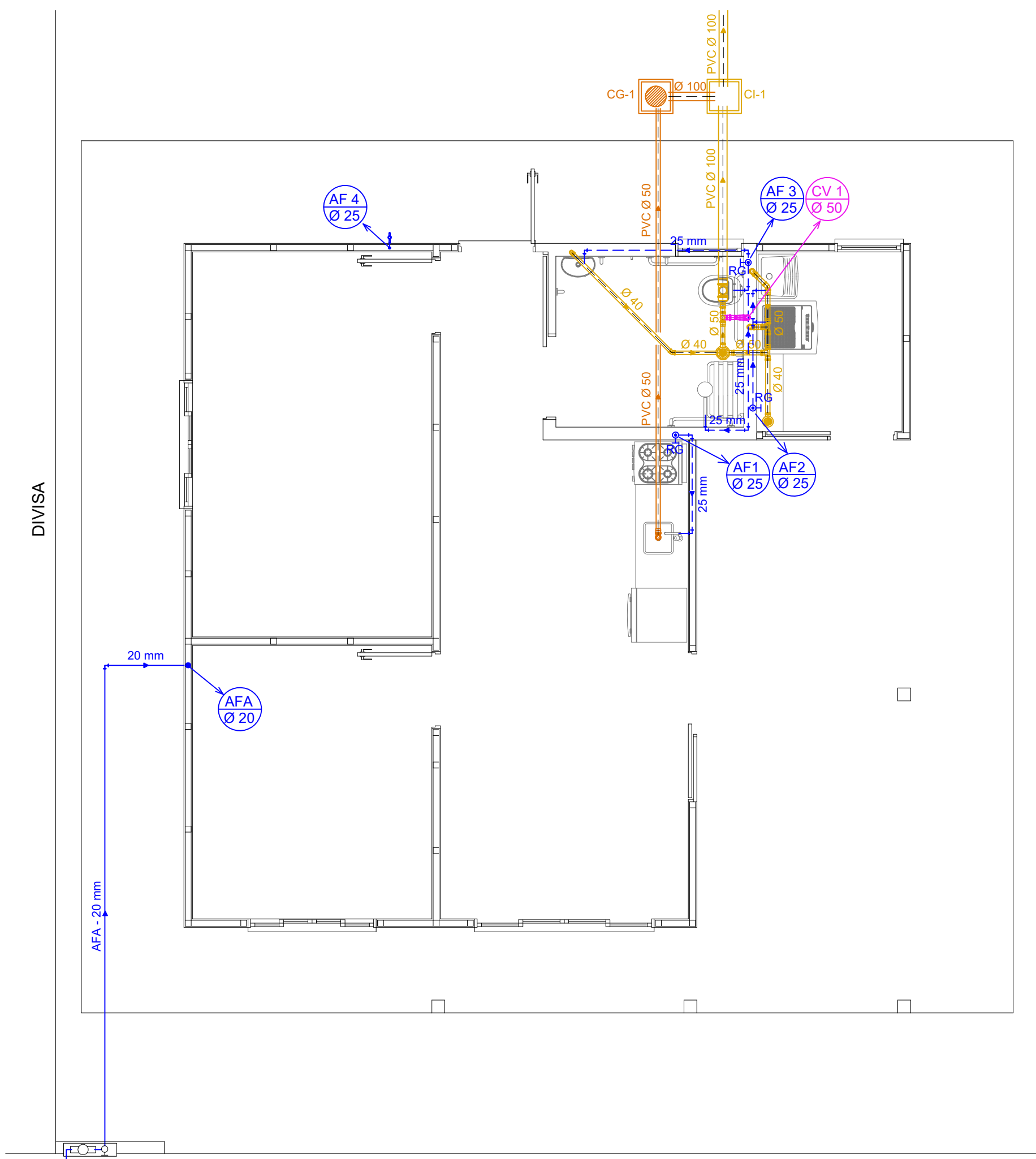
PLANTA BAIXA PAVTO. Escala 1 : 50
