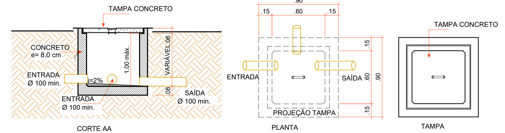
DETALHE CAIXA DE INSPEÇÃO
