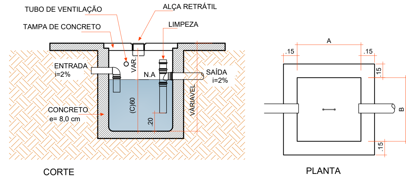
DETALHE CAIXA DE GORDURA
