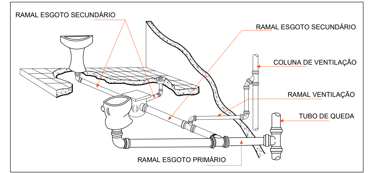
COLUNA DE VENTILAÇÃO
