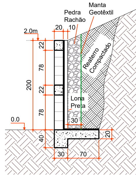
CORTE B-B
