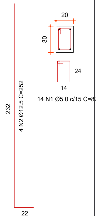
VIGA INTERMEDIÁRIA
