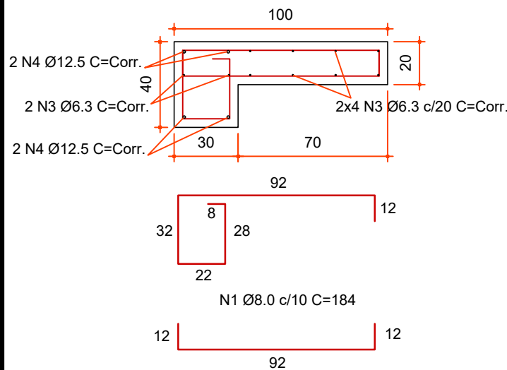
SAPATA CORRIDA
