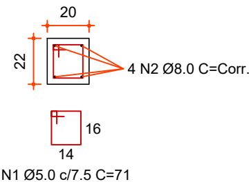
VIGA SUPERIOR
