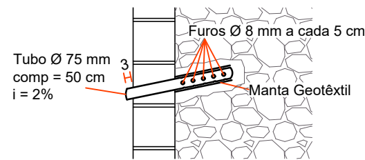
DETALHE BARBACÃ
