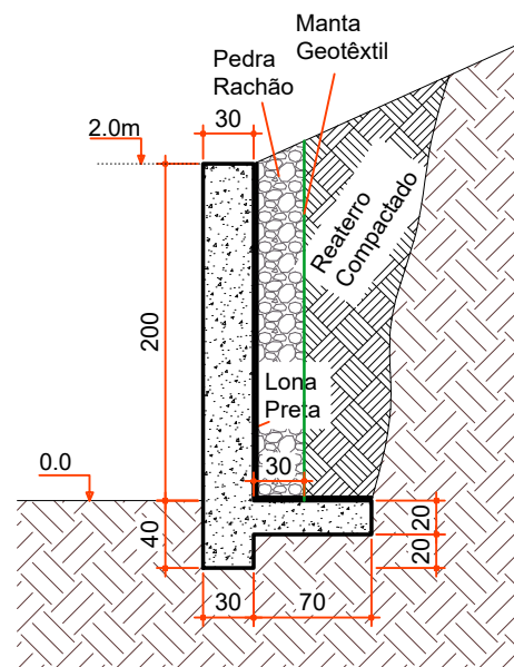
CORTE A-A
