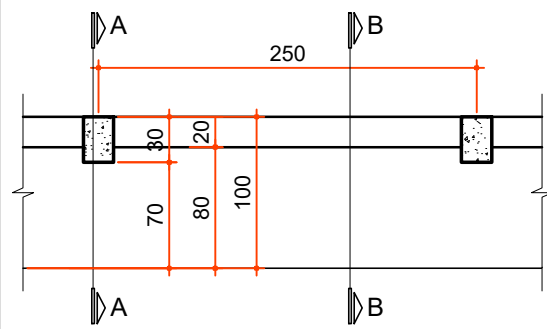
PLANTA BAIXA
