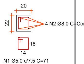
VIGA INTERMEDIÁRIA
