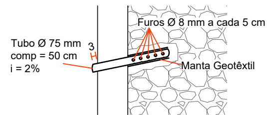
DETALHE BARBACÃ
