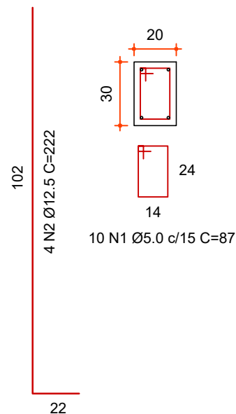
PILARES
