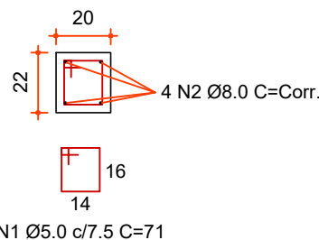
VIGA SUPERIOR
