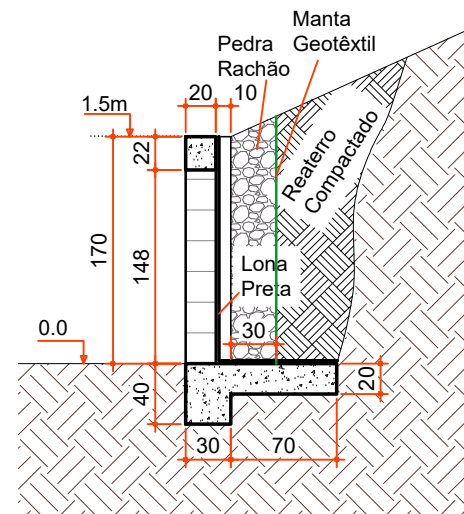
CORTE B-B
