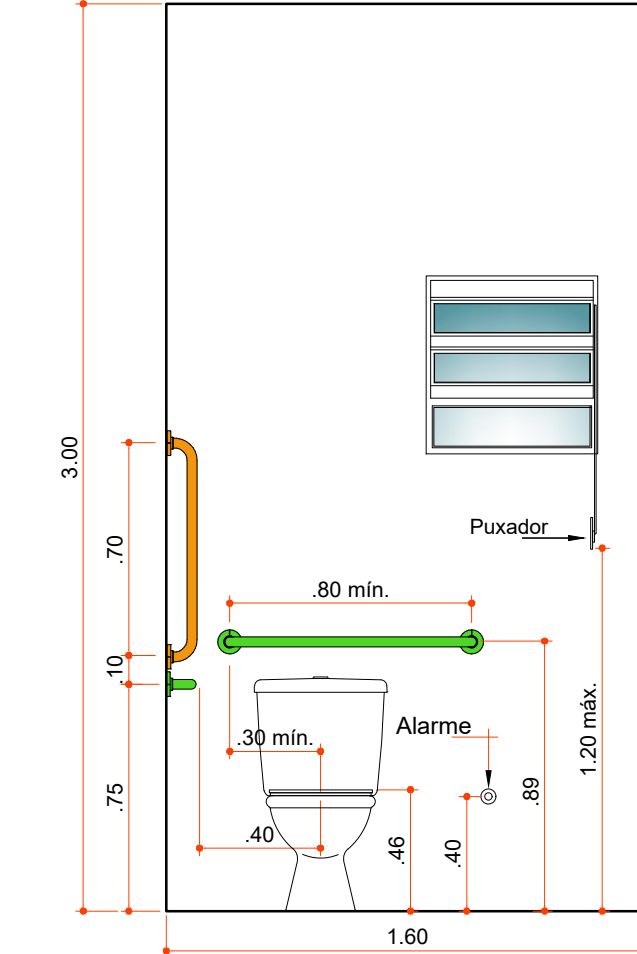
VISTA PAREDE 03
