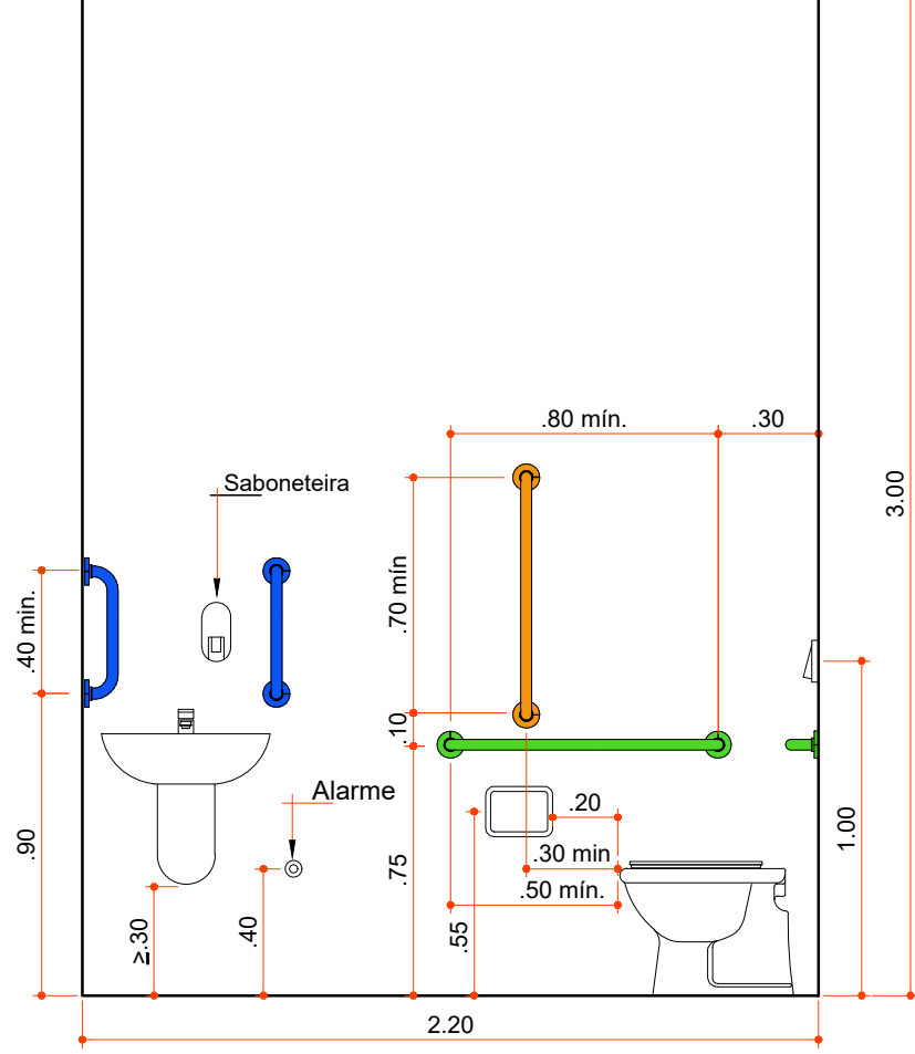
VISTA PAREDE 02
