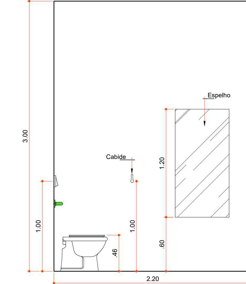
VISTA PAREDE 04
