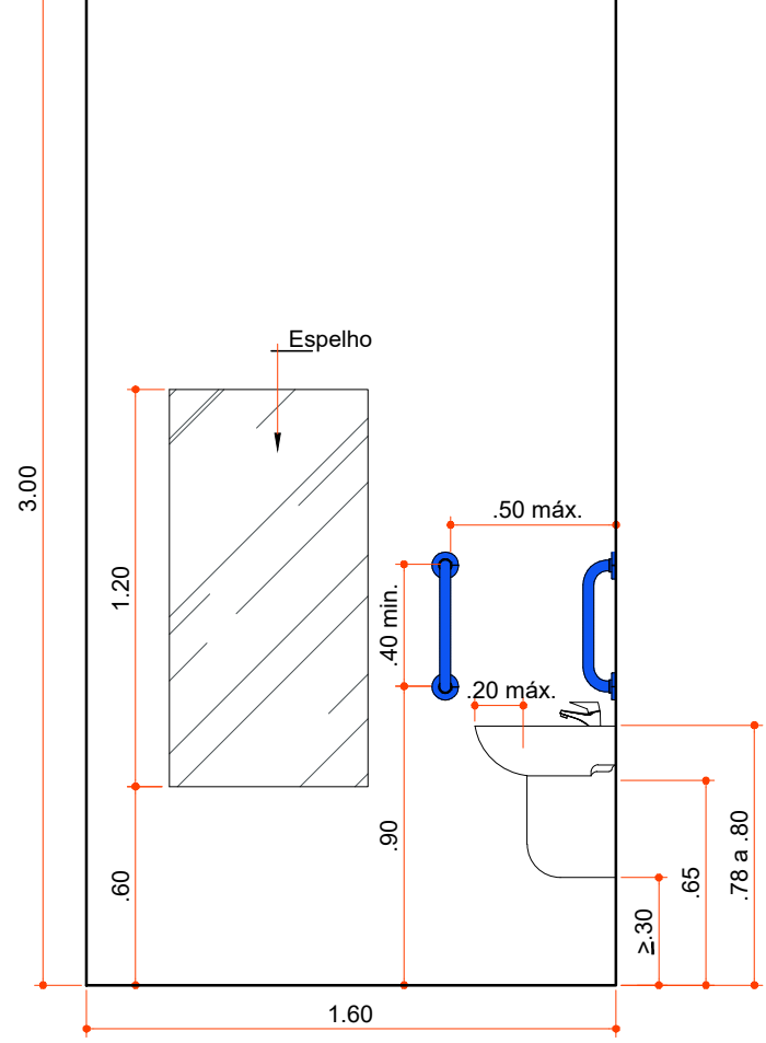
VISTA PAREDE 01
