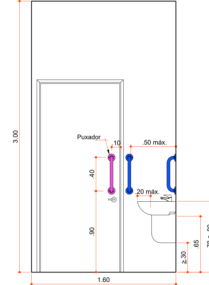
VISTA PAREDE 01
