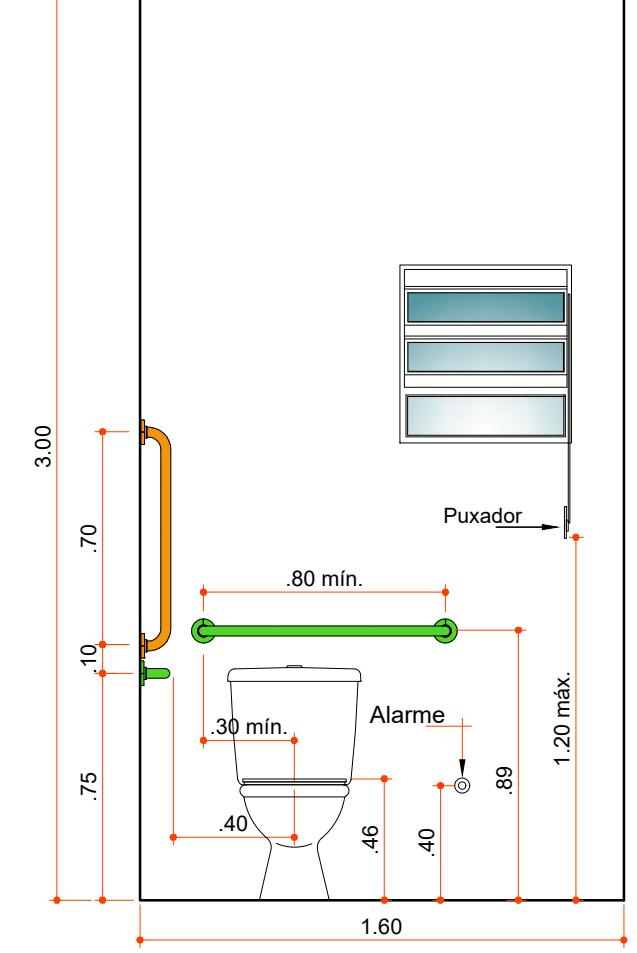
VISTA PAREDE 03
