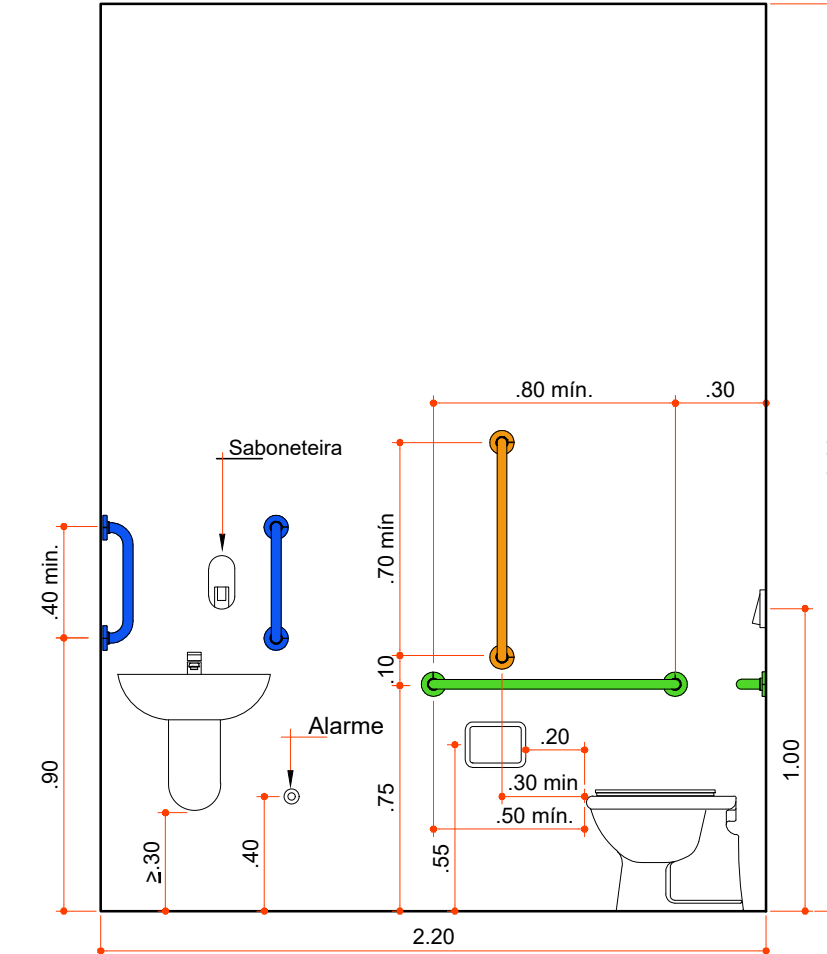
VISTA PAREDE 02
