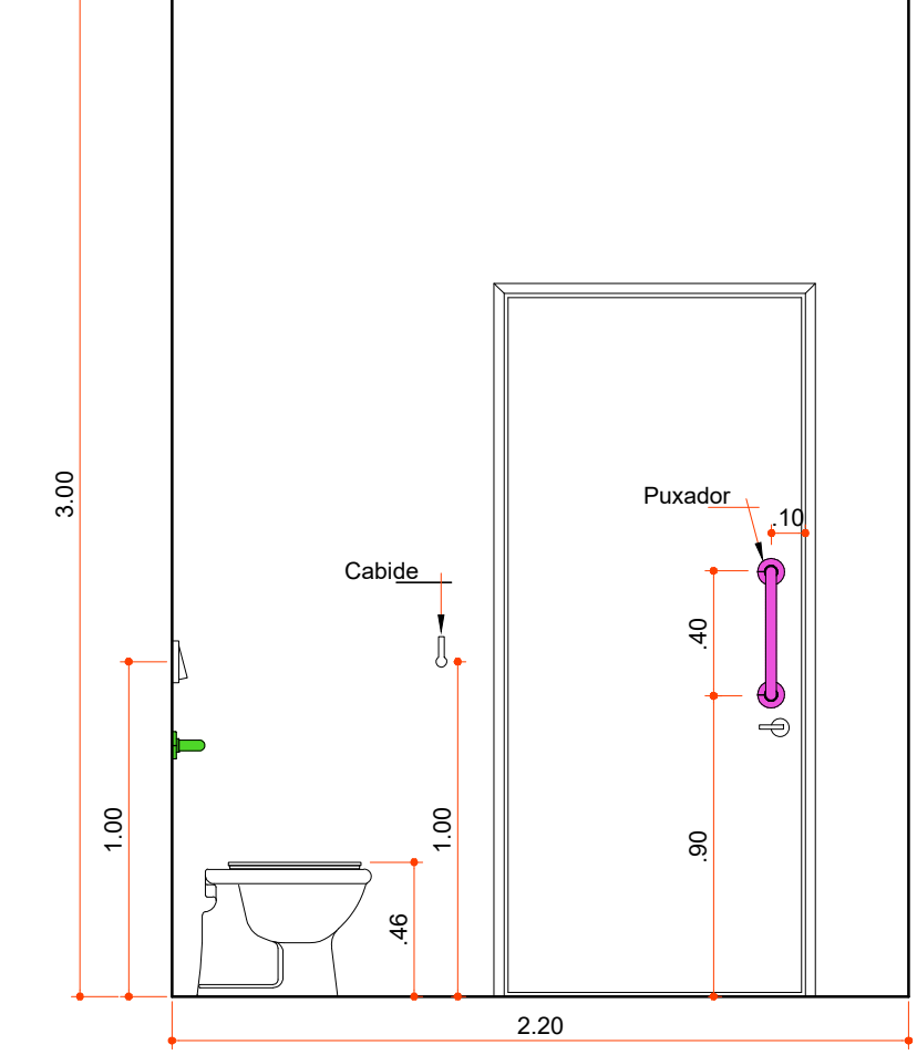
VISTA PAREDE 04
