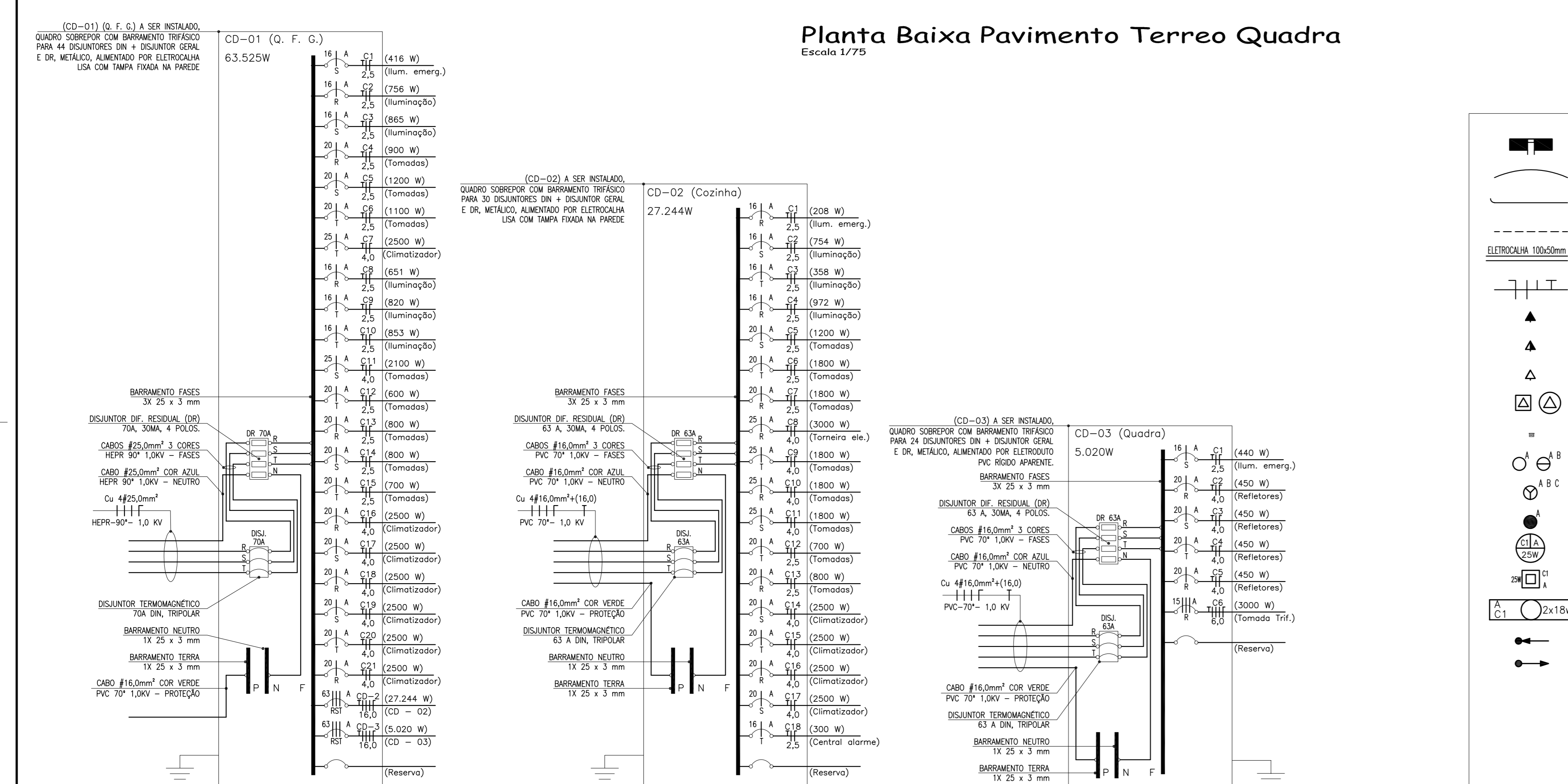
Diagrama Unifilar Quadros de Distribuição. Sem Escala
