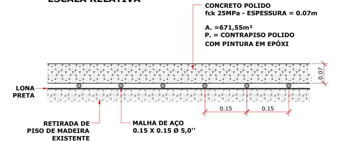
CORTE DETALHE PISO ESCALA RELATIVA
