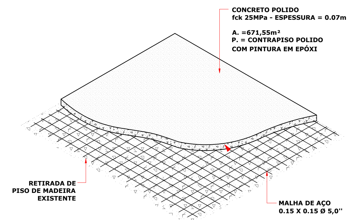
DETALHE PISO ESCALA RELATIVA
