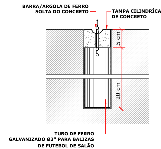
DETALHE 01 (TRAVE DE FUTSAL) ESCALA RELATIVA
