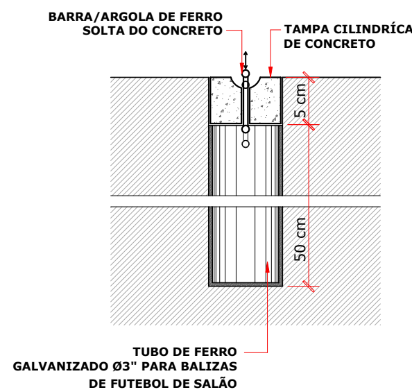
DETALHE 02 (TRAVE DE VOLEIBOL) ESCALA RELATIVA
