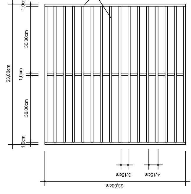
VISTA SUPERIOR DETALHE DA GRADE ESCALA:1/10
