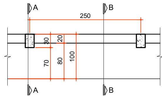
PLANTA BAIXA
