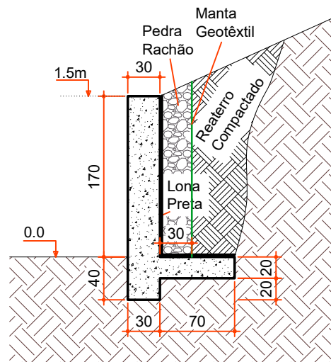
CORTE A-A
