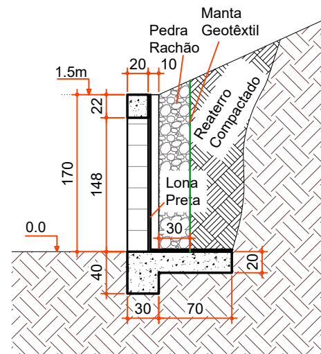
CORTE B-B
