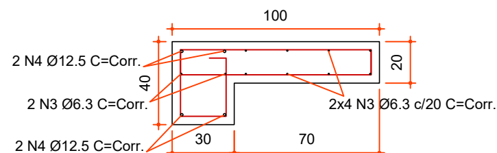
SAPATA CORRIDA
