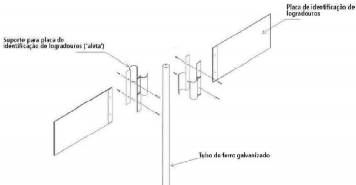
Figura 1 - Detalhe Fixação Placas
