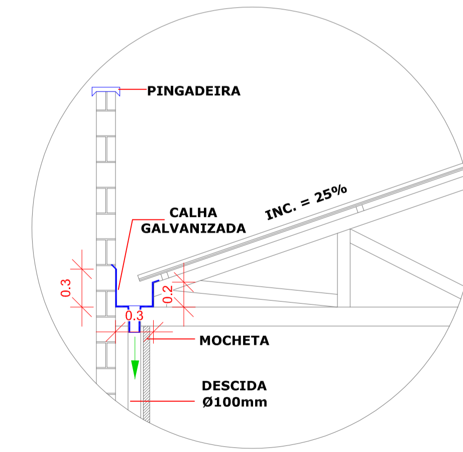
DETALHE CALHA ESCALA 1:20
