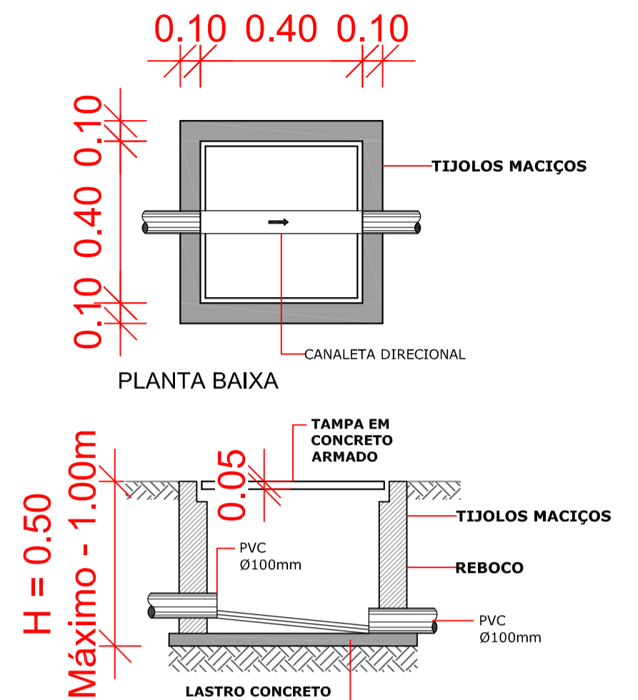
C.P. CAIXA DE PASSAGEM ÁGUAS PLUVIAIS ESCALA RELATIVA
