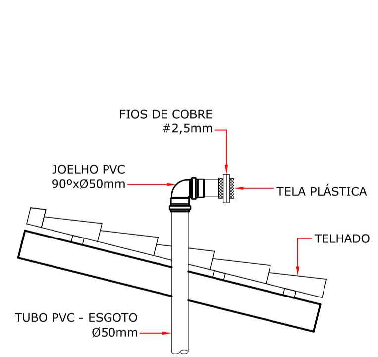
DET. DA EXTREMIDADE DA VENTILAÇÃO ESCALA RELATIVA
