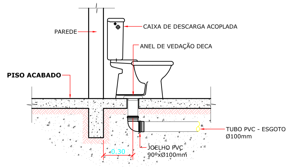
DETALHE GENÉRICO DO VASO SANITÁRIO ESCALA RELATIVA
