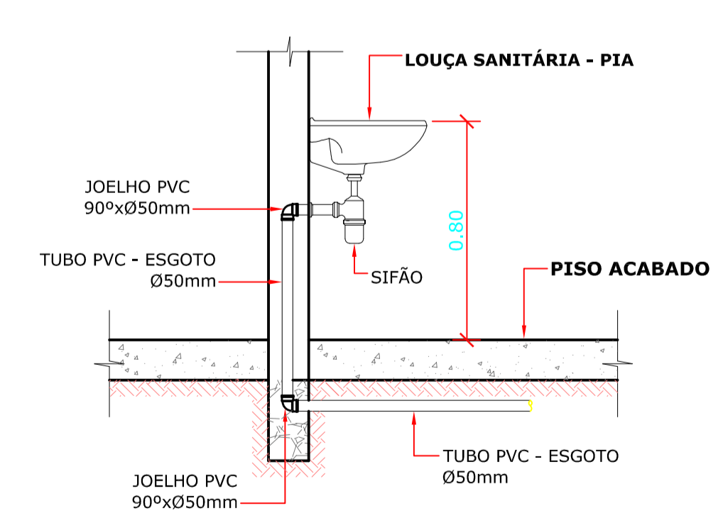
DETALHE DO LAVATÓRIO ESCALA RELATIVA
