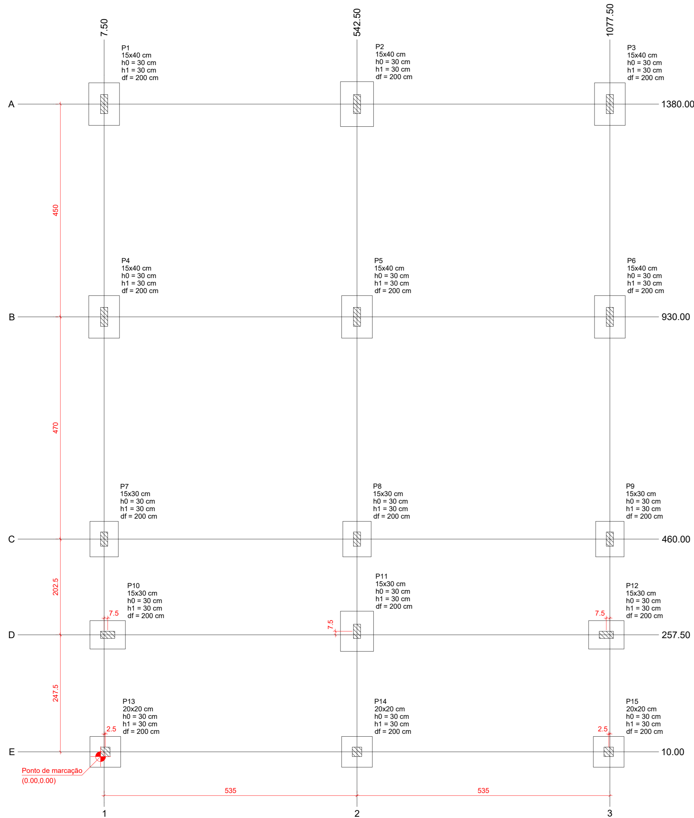
Planta de locação
