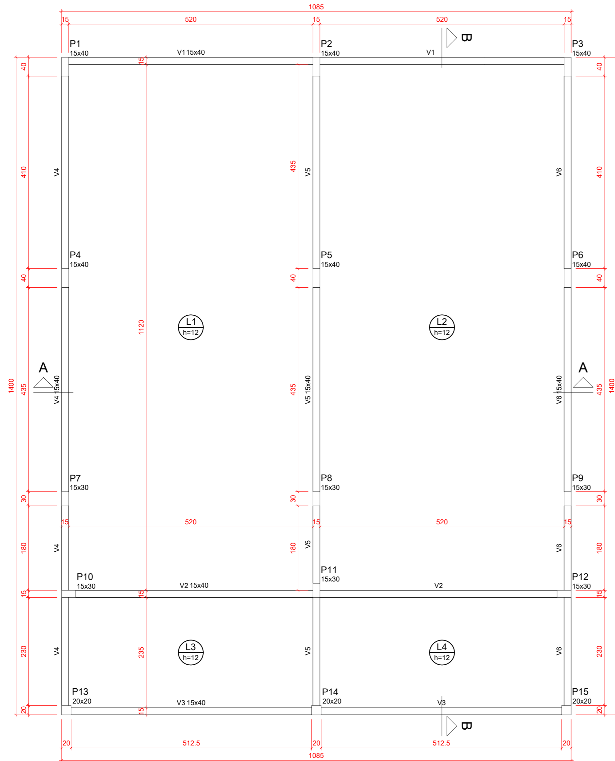
Planta de Formas do Piso (Nível 0)
