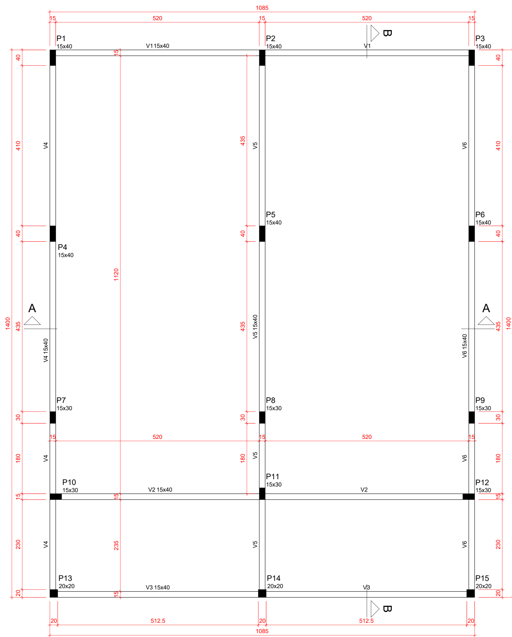
Planta de Formas da Cobertura (Nível 350) escala 1:50
